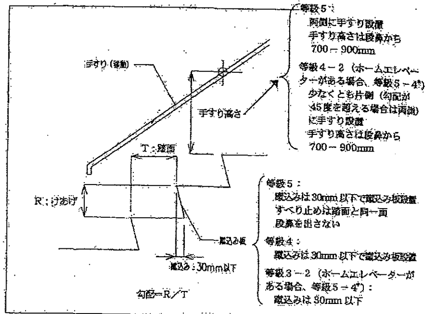
図9-7 階段のディテール
