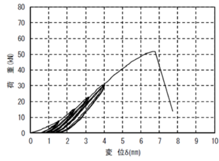
試験体記号 S-NU-K
