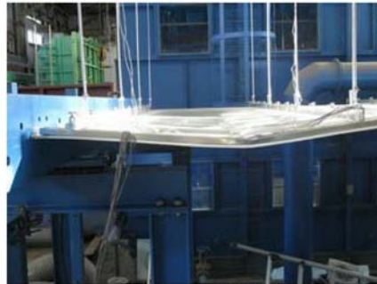
写真 1.1.4 破壊状況 天井面材及び野縁の座屈
