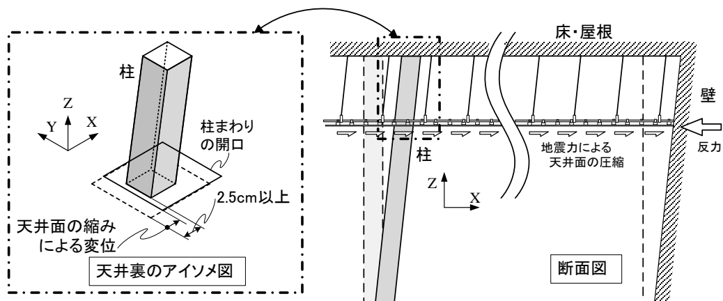
図 18 柱まわりの強制変位と天井面の縮みによる変位
