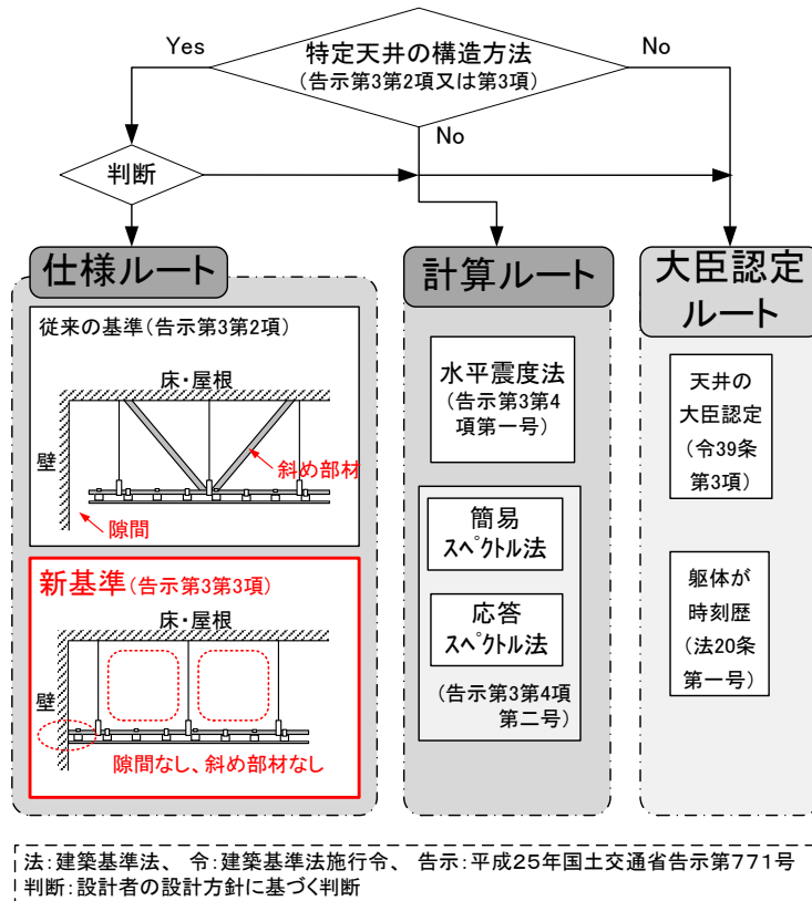
図 1 新基準の位置付け
