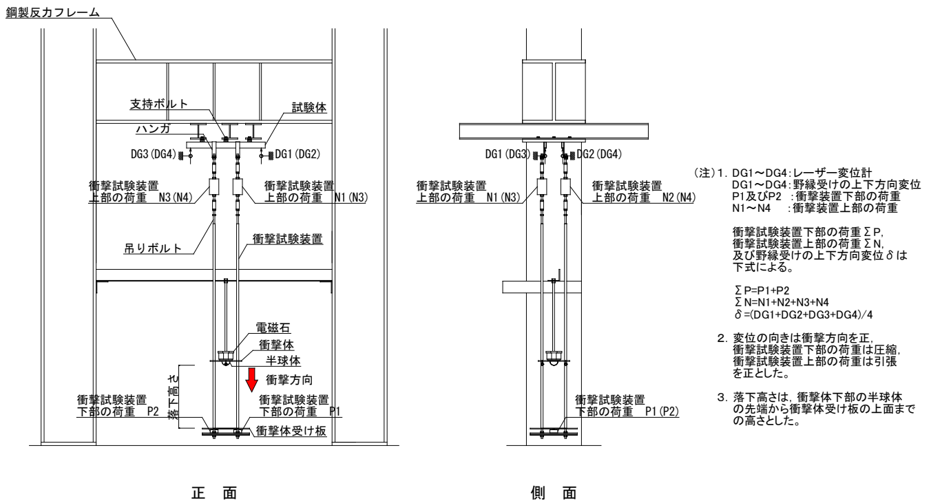
図 24 試験方法 (例) 天井面法線方向
