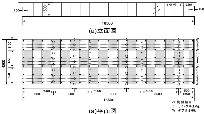
図 45 大規模試験体 12)
