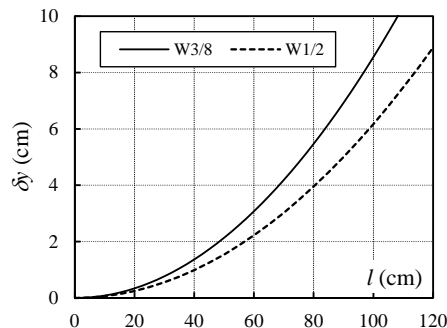
図 43 弾性限の水平変位 \delta_y
