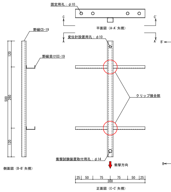
図 19 試験体 (例) 野縁方向試験体
