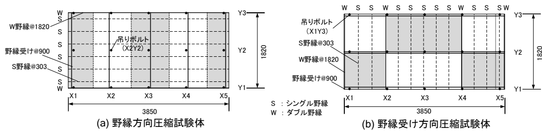
図 44 小規模試験体 12)
