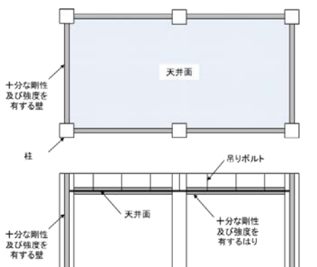
図 15 天井面周囲の壁やはり
