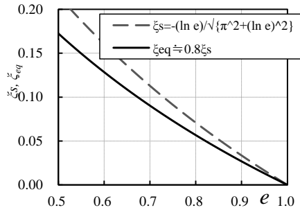
図 35 e と \xi_s 及び \xi_{eq} との関係
