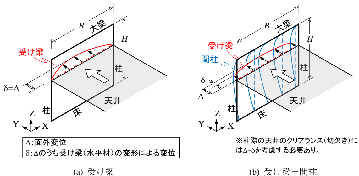
図 40 変形制限
