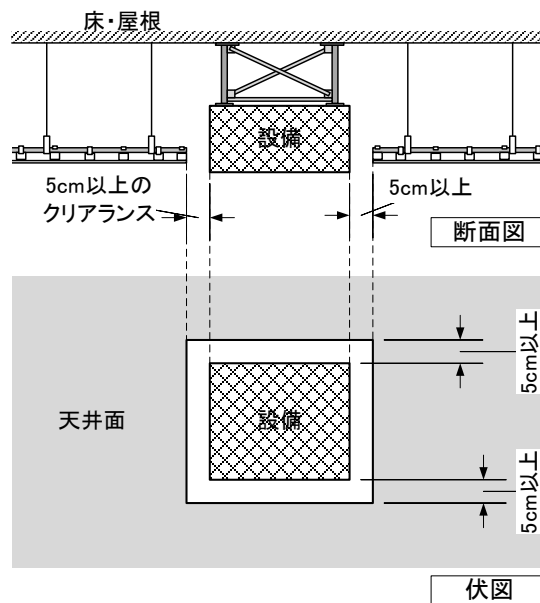
図 17 設備等とのクリアランス
