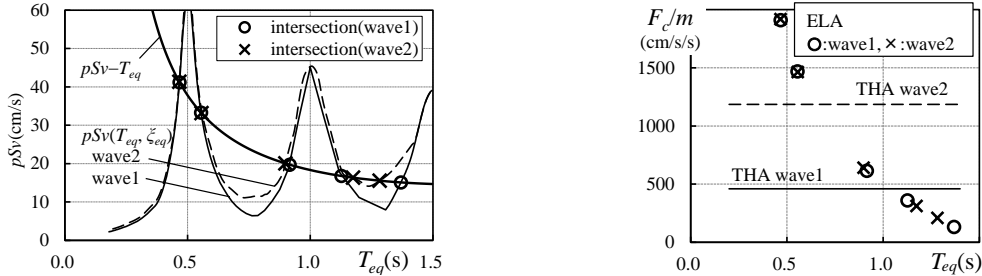
(a) 多峰形の床応答スペクトルになる 2 つ入力波に (b) 衝撃力の評価 (図(a)の交点に対応する等価線形化法に対する等価線形化法の複数の解 化法の解。THA は時刻歴応答解析)
