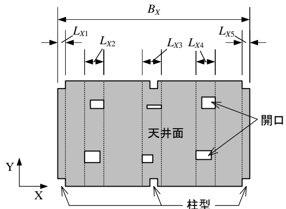
図 13 幅開口率（柱型がある場合）
