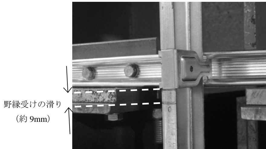
写真 3 野縁受け方向の試験実施例
