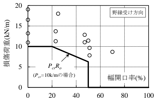
図 14 幅開口率と損傷荷重の関係 文献 12)13)14) のデータを基に作成
