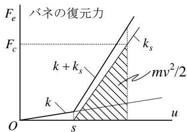
図 31 最大速度 v による衝撃力 F_c
