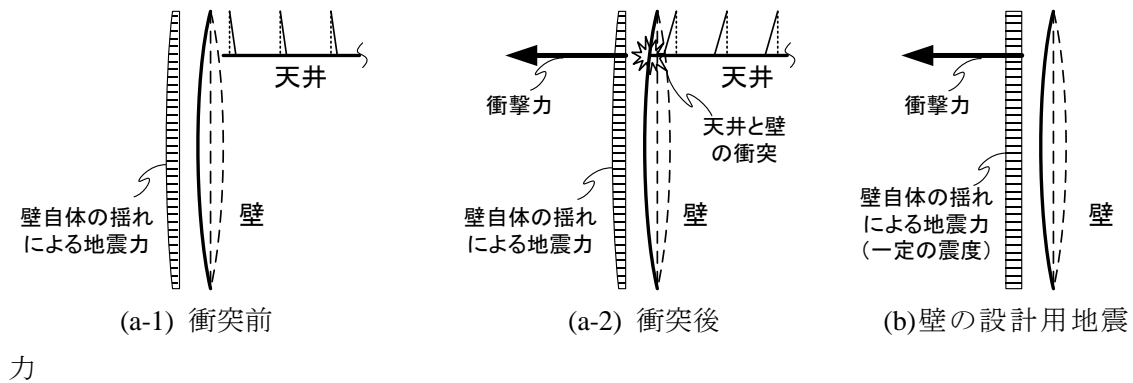
図 39 壁の設計用震度（壁際の断面図と壁の地震力）
