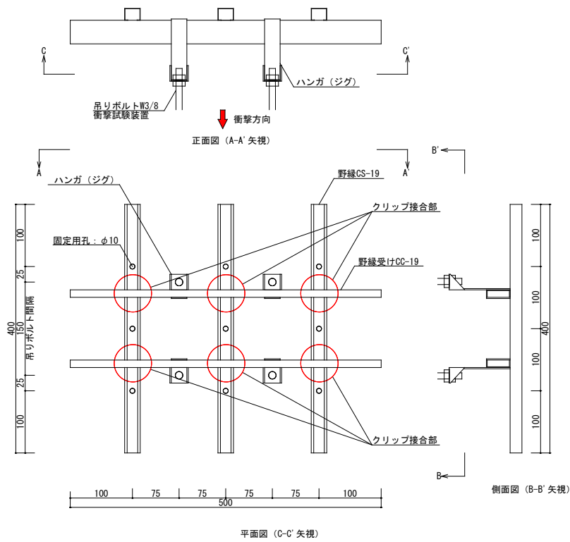
図 21 試験体 (例) 天井面法線方向試験体
