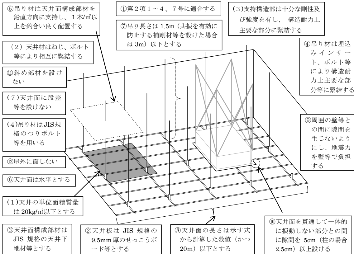
図 3 技術基準の概要（（ ）数字は第 2 項、丸数字は第 3 項による）
