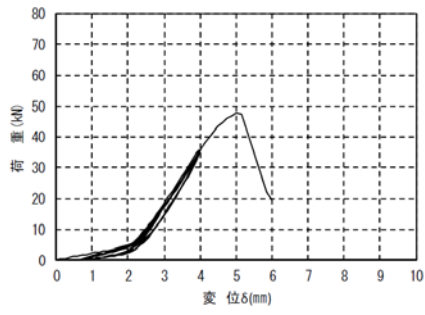
試験体記号：K-NU-K
