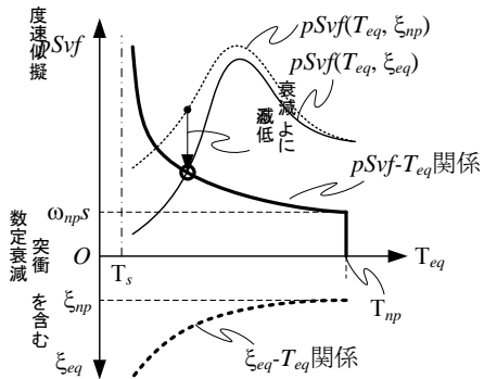
図28 等価線形化法 3) の概要 pSvf \sim T_{eq} 関係（イメージ）
