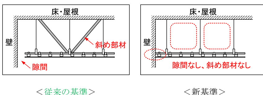
図1 従来の基準と新基準（壁際の断面図）
