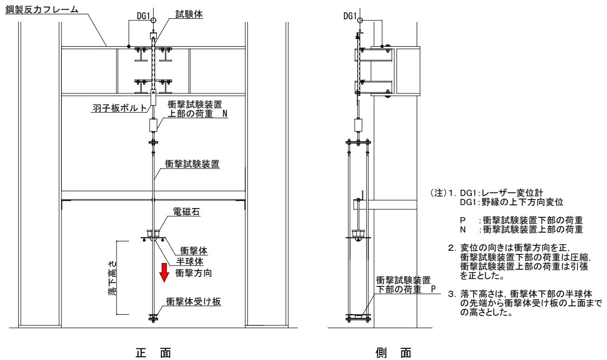
図 22 試験方法 (例) 野縁方向
