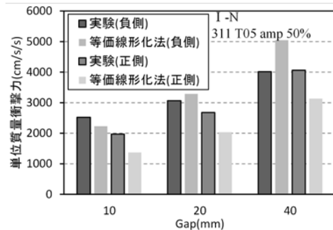
図29 衝撃力の推定（等価線形化法）
