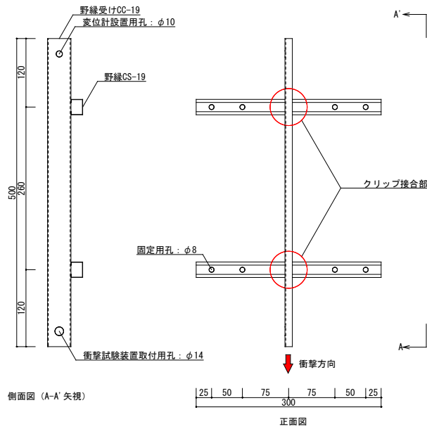
図 20 試験体 (例) 野縁受け方向試験体
