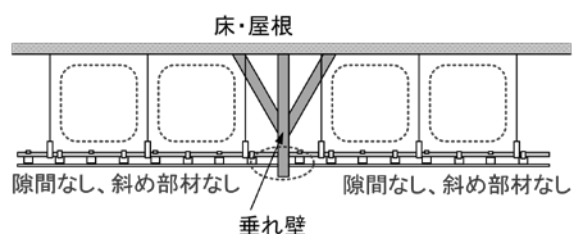
図 16 天井の間にある垂れ壁
