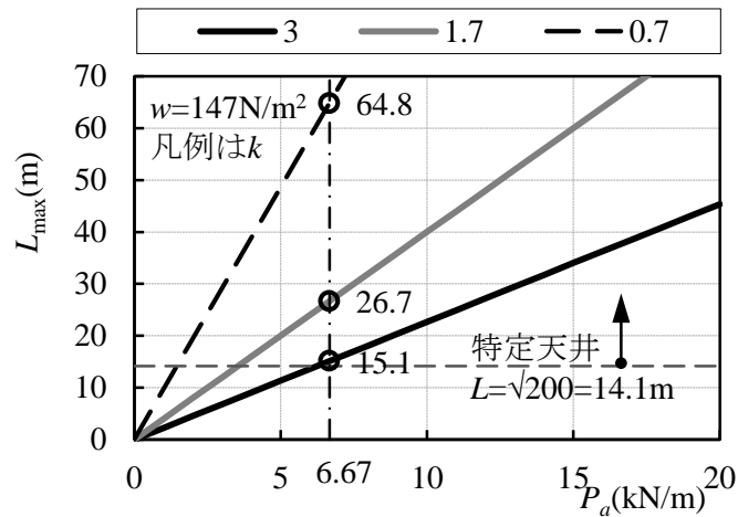
図 A 1 許容耐力と天井長さの関係
