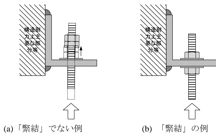
図 6 吊り材の緊結
