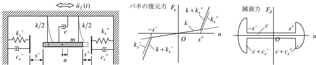
図27 1自由度衝突系
