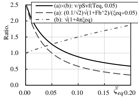
図 33 v/pSvf(T_{eq}, 0.05) （共振点）
