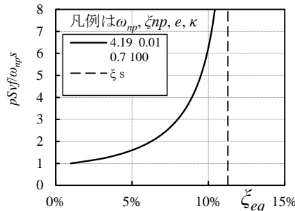
図 34 \xi_{eq} の変化の例（ 2\pi/\omega_{np}=1.5 (s)、 \xi_{np}=0.01 、 e=0.7 、 \kappa=100 ）
