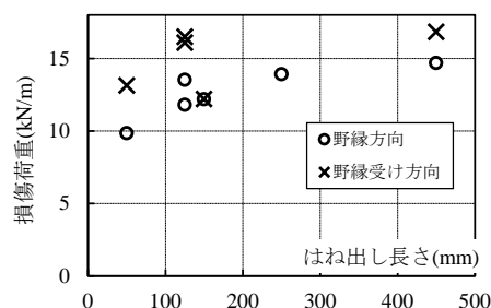
図 8 はね出し長さと損傷荷重の関係（面内圧縮試験） 9)
