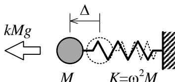
図 41 1 質点 1 自由度系
