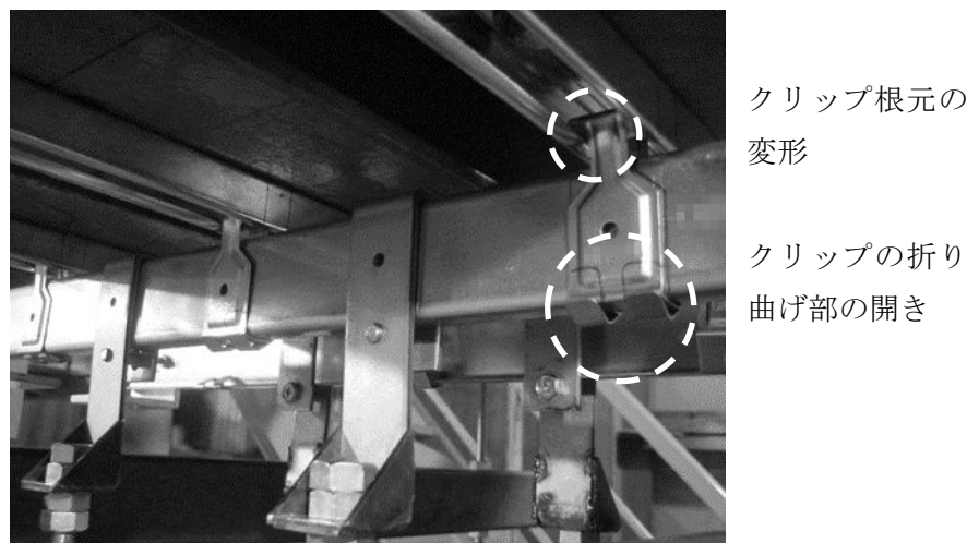
写真 4 天井面法線方向の試験実施例
