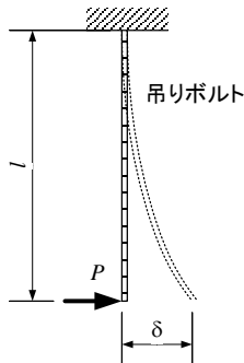
図 42 吊りボルト
