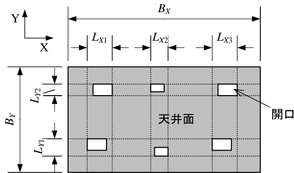
図 12 幅開口率
