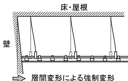
図5 吊りボルトの柔性による追従性（壁際の断面図）
