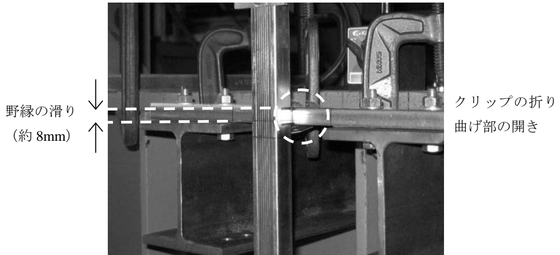
写真 2 野縁方向の試験実施例
