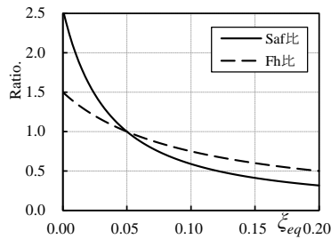
図 32 Fh 比 (式(9)) と Saf 比 (式(11)) の比較
