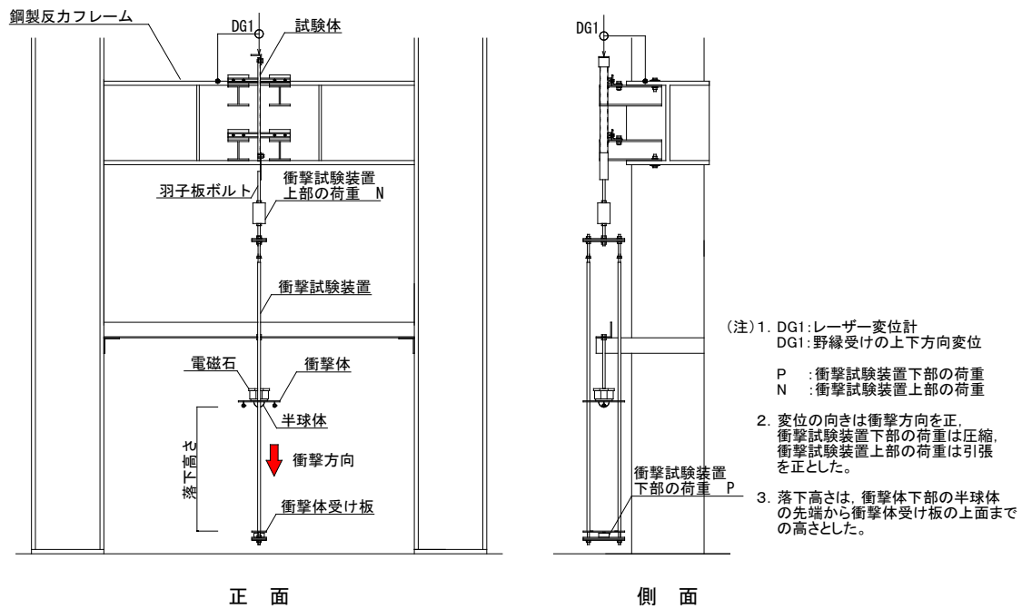
図 23 試験方法 (例) 野縁受け方向
