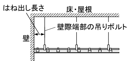
図 7 はね出し長さ（壁際の断面図）
