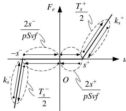
図 38 \Delta t^\pm の近似式の構成
