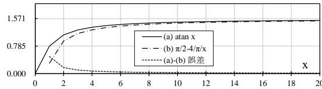
図 37 \tan^{-1}x \approx \pi/2 - 4/(\pi x)
