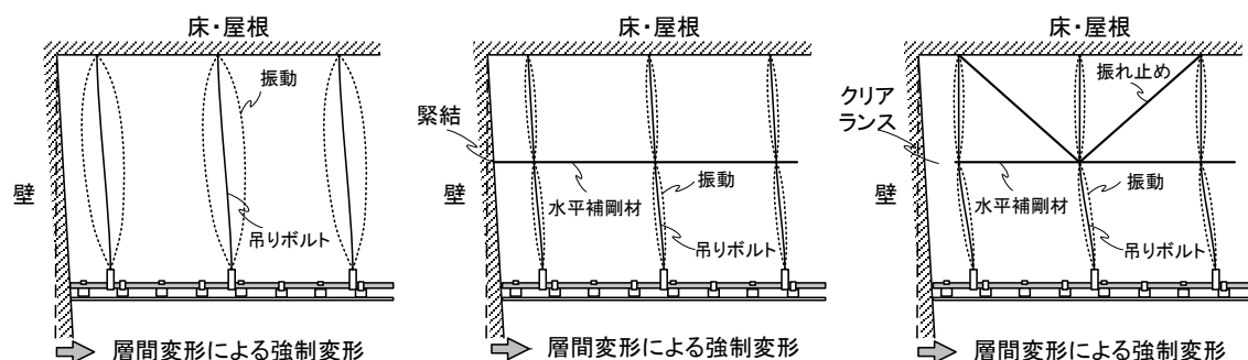
(a) 水平補剛材なし (b) 水平補剛材あり(緊結) (c) 水平補剛材あり(振れ止め)
