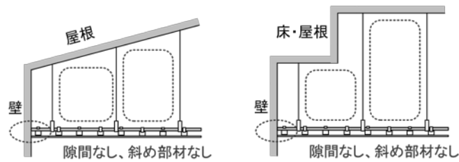
図 10 吊り長さが変化する／異なる場合
